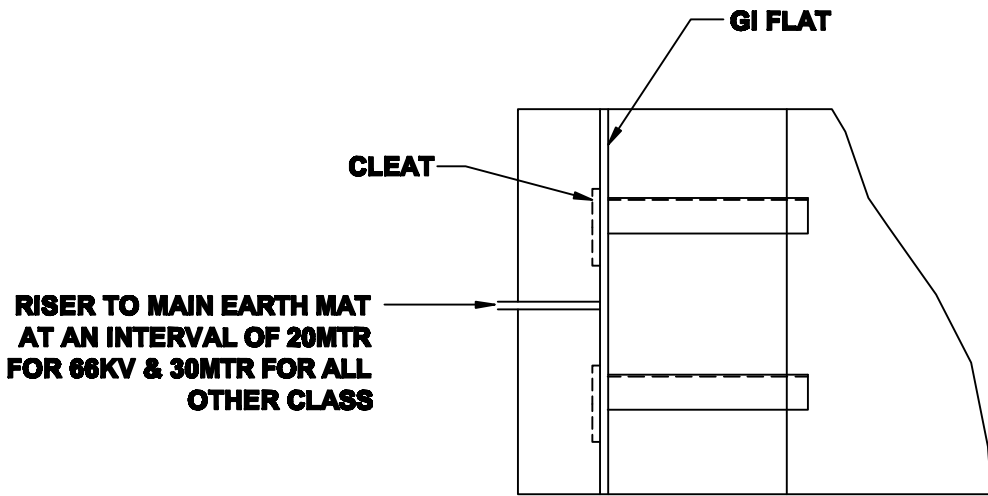
TYP. PLAN
